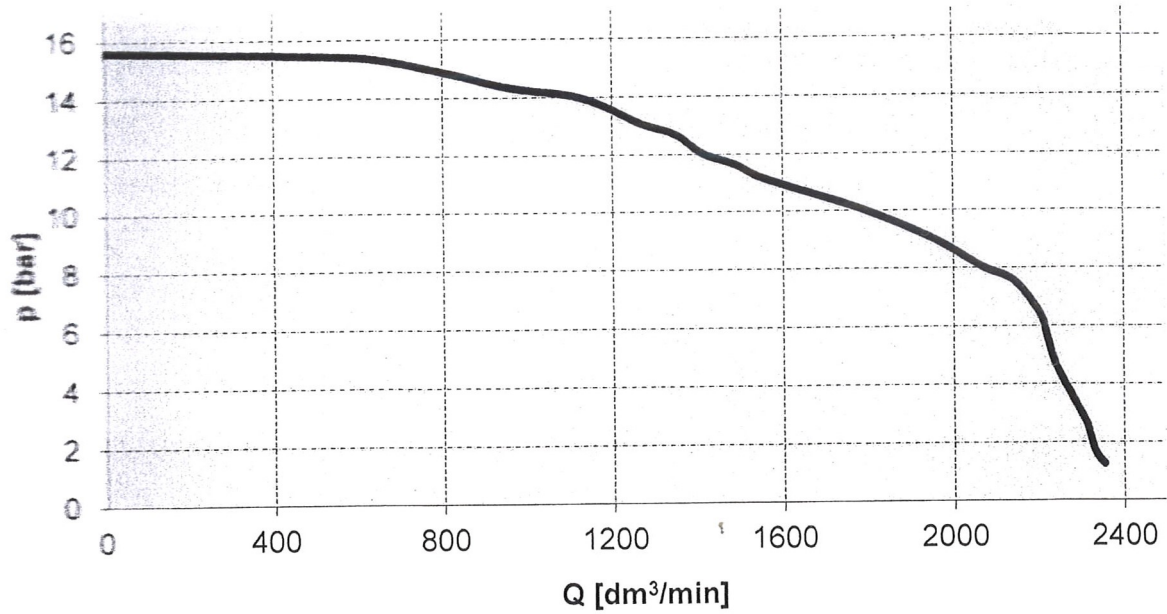
Rys. 1. Charakterystyka motopompy dla H gs =1,5 m
