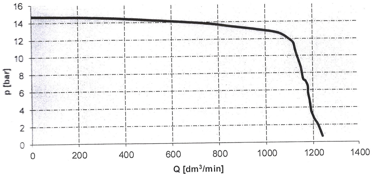
Rys. 2. Charakterystyka autopompy dla H gs =7,5 m
